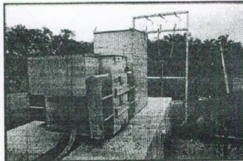
CÁRCAMO 4 DE AGUAS NEGRAS 12 JULIO 2010
